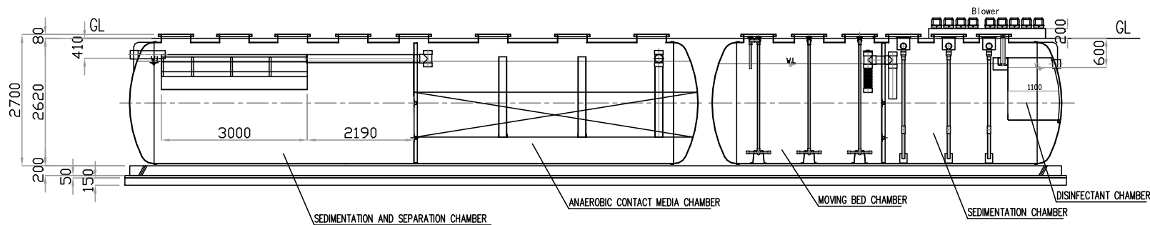
A-A SECTION
