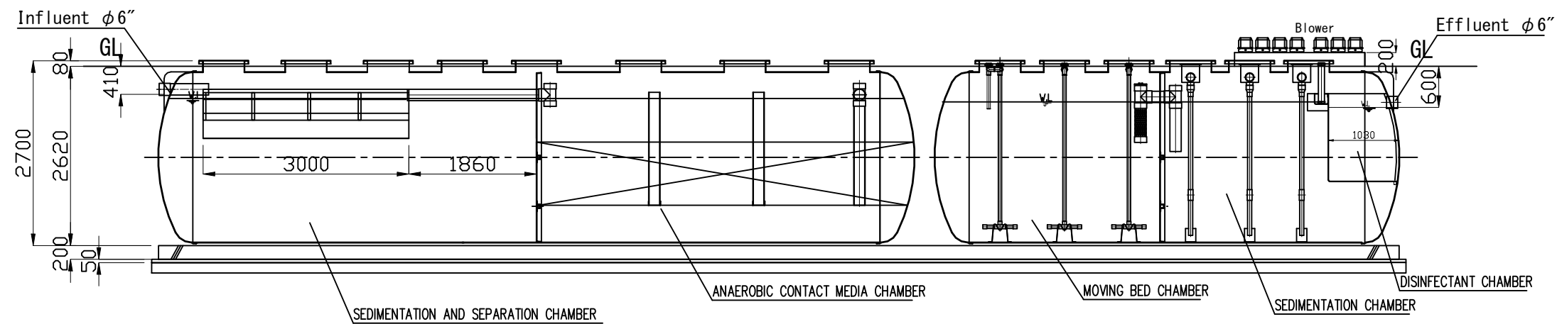
A-A SECTION
