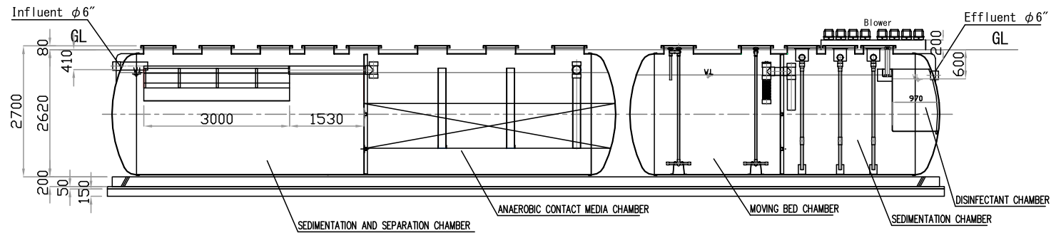
A-A SECTION
