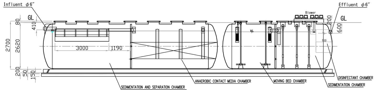
A-A SECTION
