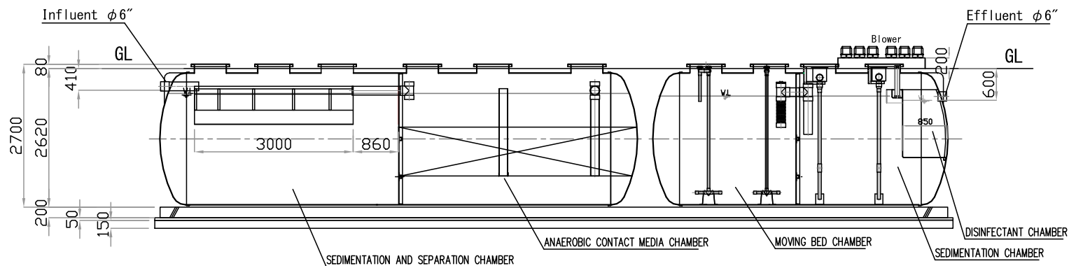
A-A SECTION
