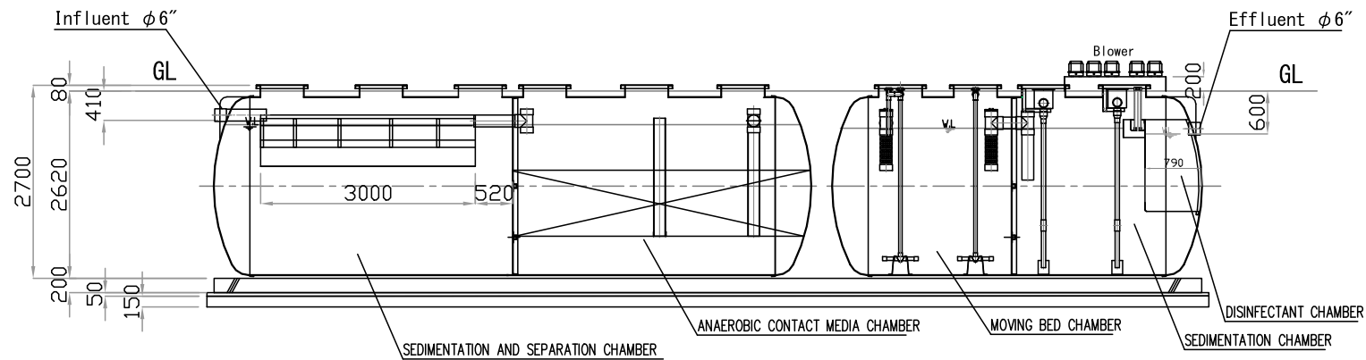
A-A SECTION
