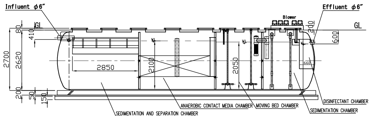
A-A SECTION
