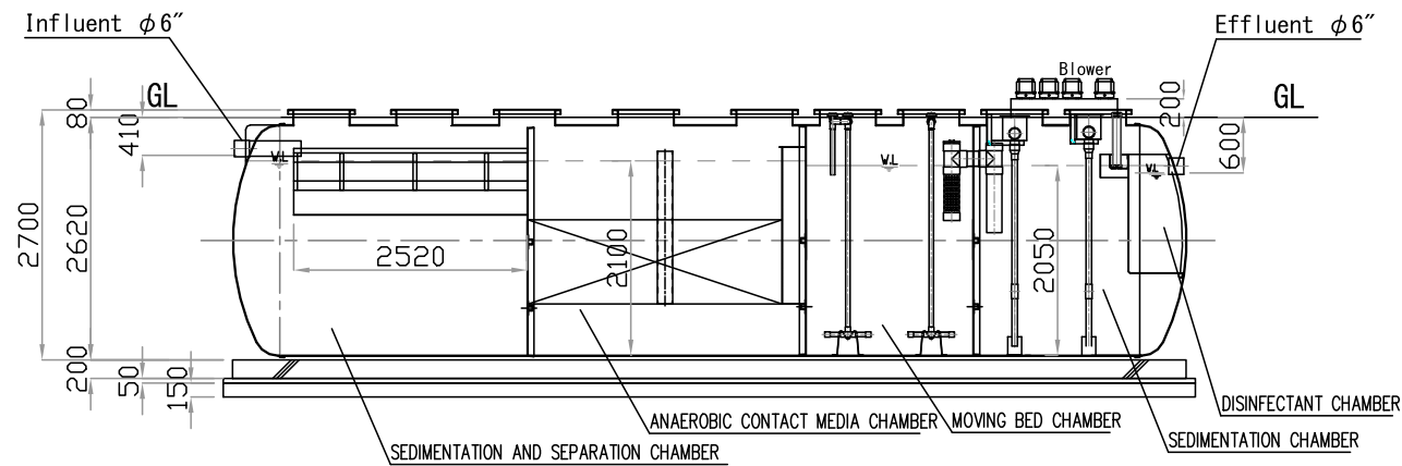
A-A SECTION
