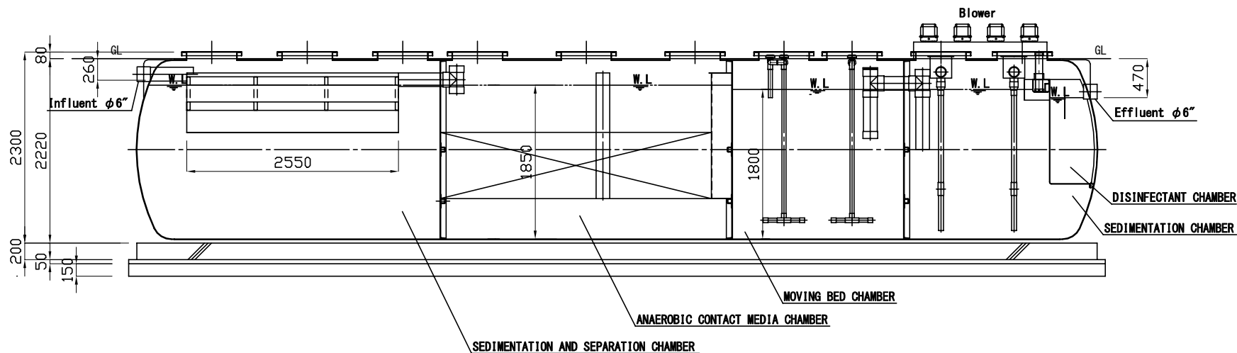
A-A SECTION
