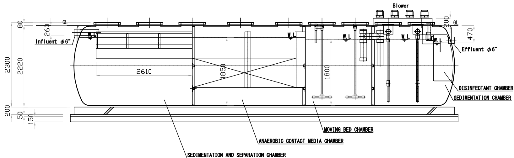
A-A SECTION
