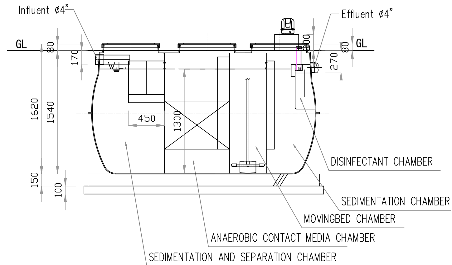
A-A SECTION
