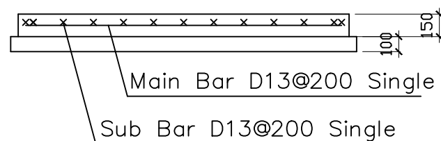
A-A SECTION
