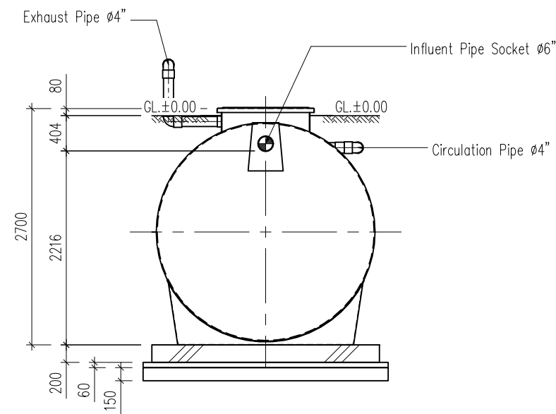
B - B SECTION NTS=====
