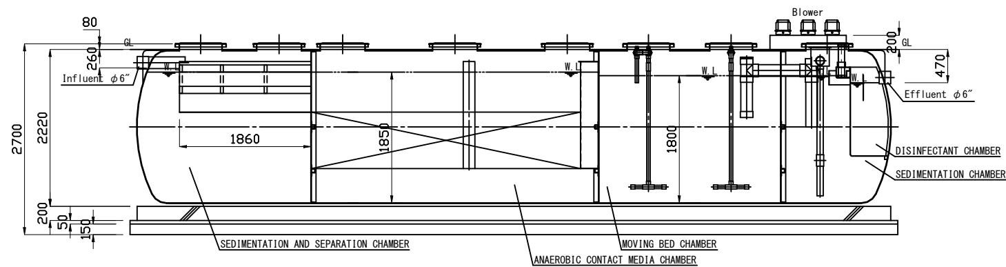
A-A SECTION
