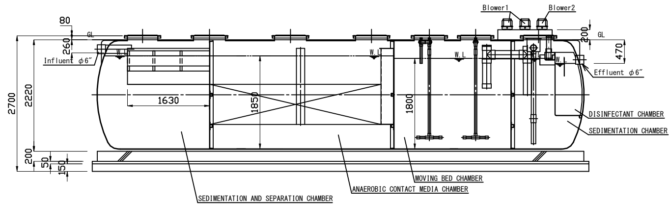
A-A SECTION
