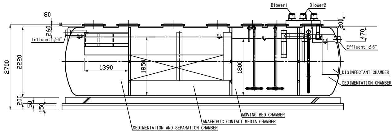
A-A SECTION
