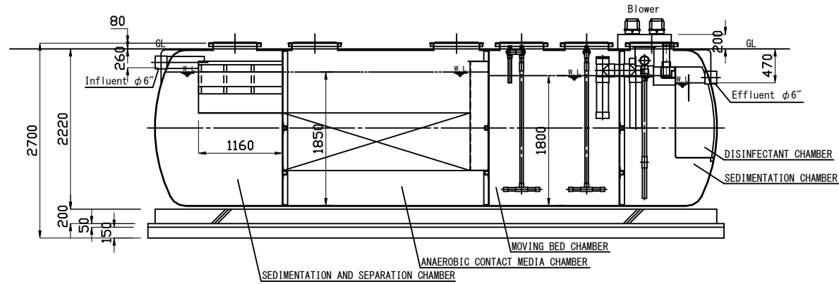
A-A SECTION
