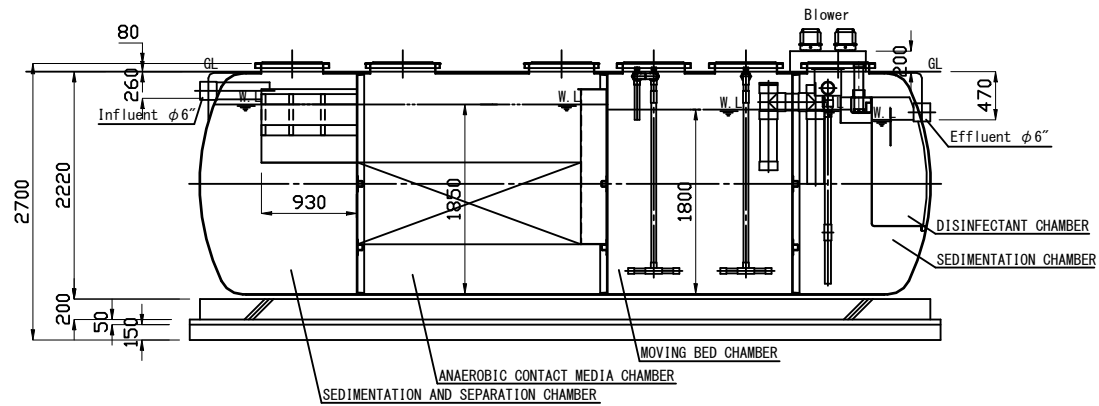
A-A SECTION
