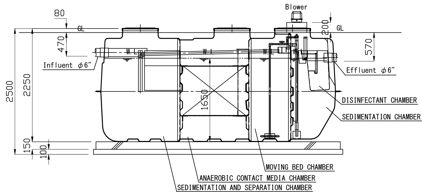
A-A SECTION
